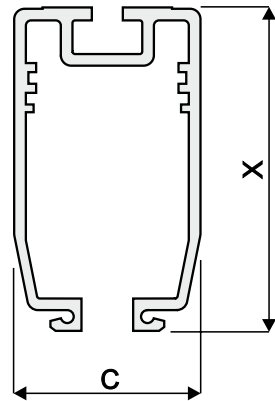
SPR 85, SPR 125, SPR 160A
